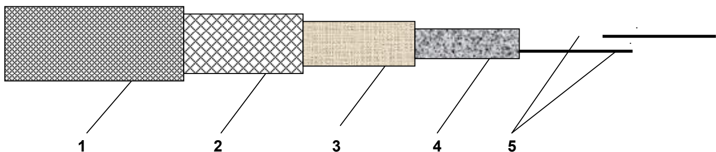
Рис. 3. Устройство нагревательного кабеля Devi-Pipeheat™ DPH-10 .
